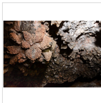
Кальцит
