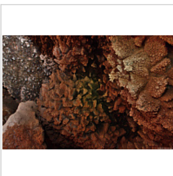
Друзы
