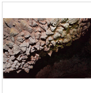
Кристаллы кальцита
