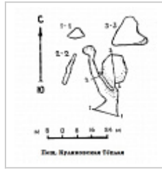
Пещ. Куликовская Тёплая (план и разрезы) Печеркин И.А., Матарзин Ю.М., Карзенков Г.И., Мацкевич И.К., 1963 г.
