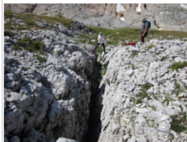
Вход пещеры Василиса, А.Ю.Рычагов измеряет азимут трещины
