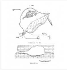
Пещ. Жёлтый грот (план и разрезы) Панарина Г.Н., 1968 г.
