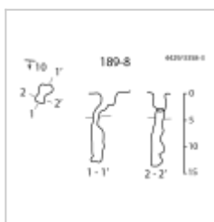
189-8 План и разрез
