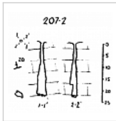
207-2 План и разрез
