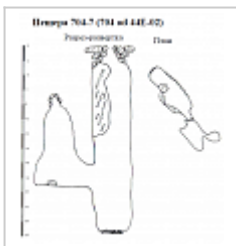
План и разрез ск Мория
