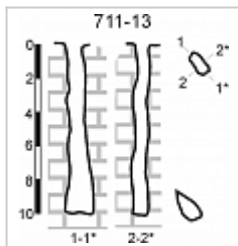
План и разрез Съемка УСА, Касьян Ю.
