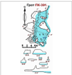
ПК 391 план и разрез
