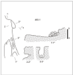
Ак-Кая 50 план и разрез
