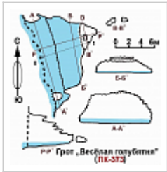
Веселая голубятня План и разрез. Пронин К.
