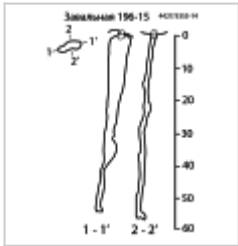
Завальная План и разрезы
