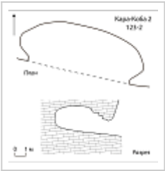
Кара-Коба 2 план и разрез
