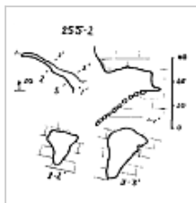
Мисхорский грот План и разрез
