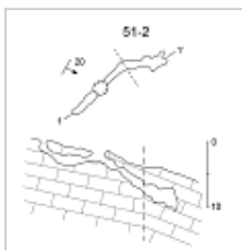
Партизанская-2 План и разрез
