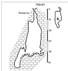
План и разрез Съёмка УСА
