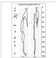
Севастопольская Разрезы и сечения
