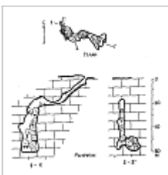
План и разрез Съёмка ККЭ
