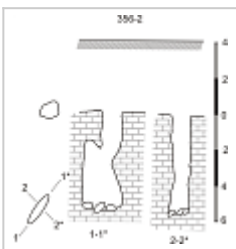
Фонтаны План и разрез
