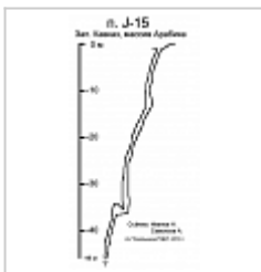
Разрез-развёртка Съёмка с/к "Сокольники- РУДН", 2010 г.
